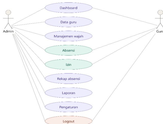
Gambar 2 Usecase Sistem
