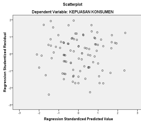
Gambar 2 grafik scatterplot
