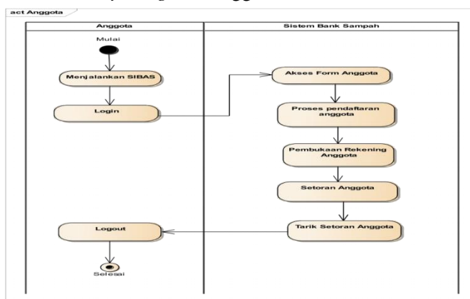
Gbr, 4 Activity Diagram Anggota
