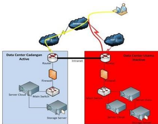
Gambar 5 Kondisi DCU mengalami gangguan(DRC menggantikan operasi DCU)
